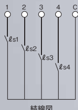
結線図
