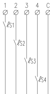
結線図
