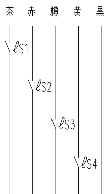
結線図
