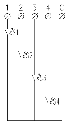
結線図
