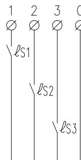
結線図
