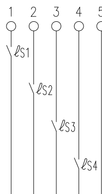
結線図
