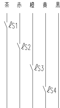
結線図
