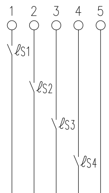
結線図
